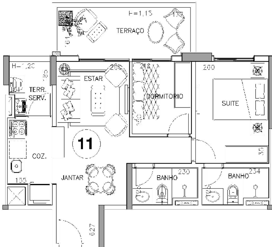
Planta tipo 60m 2
